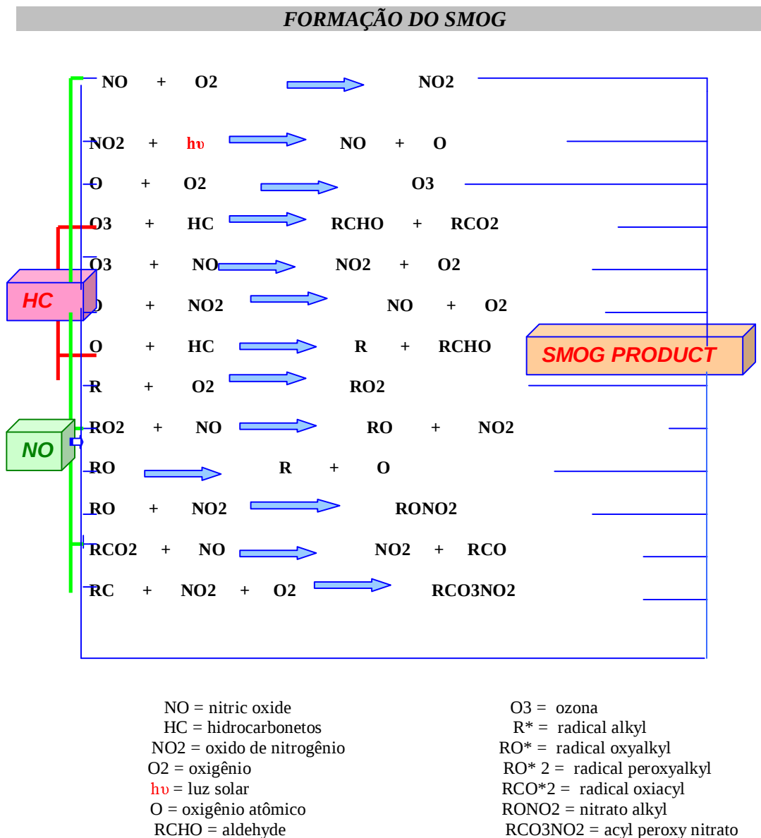
FIGURA 15 – Mecanismos generalizados das reações fotoquímicas (PERKINS, 1974).
