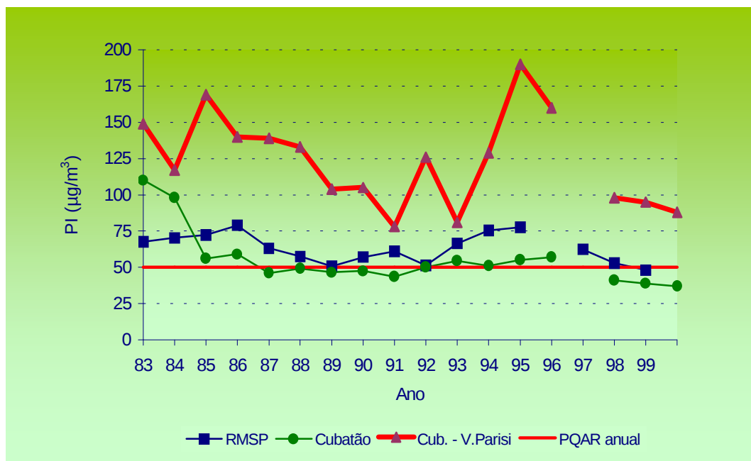
FIGURA 17 – Concentração de poeiras inaláveis (CETESB, 2000 a ).
