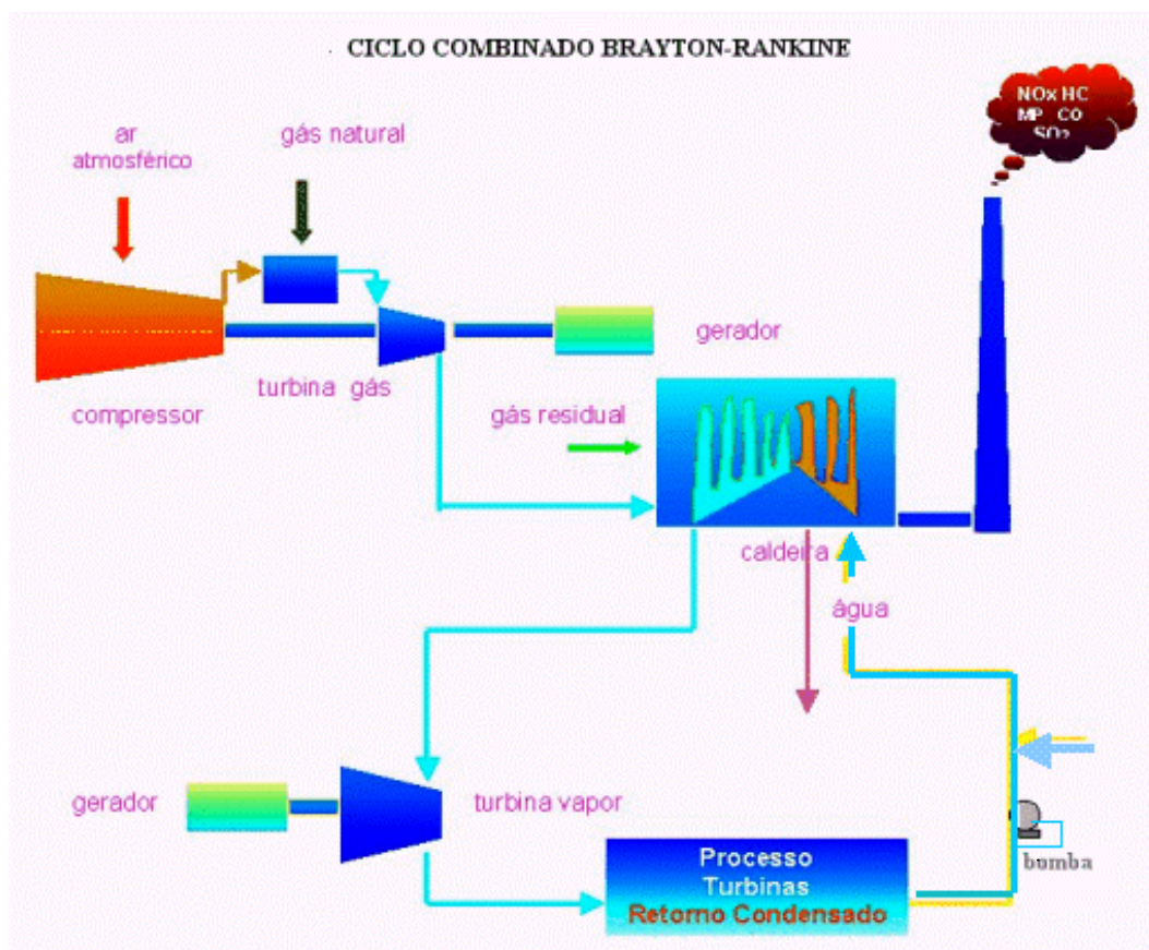
FIGURA 19 – Ciclo de geração de energia (adaptado do EIA/ RIMA CCBS, 2000).
