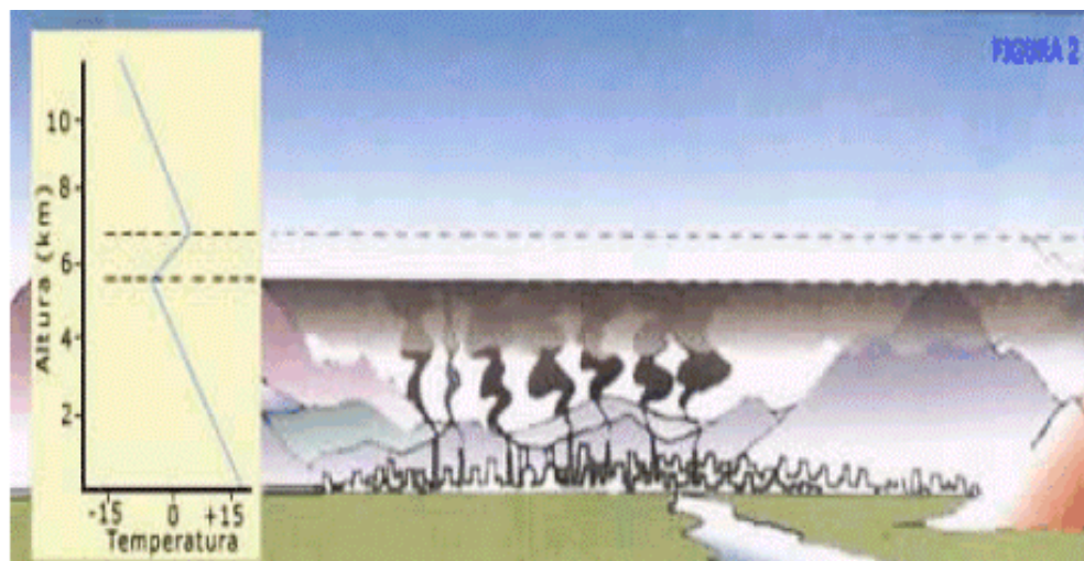
FIGURA 2 – Situação desfavorável à dispersão de poluentes (CETESB, 2003)
